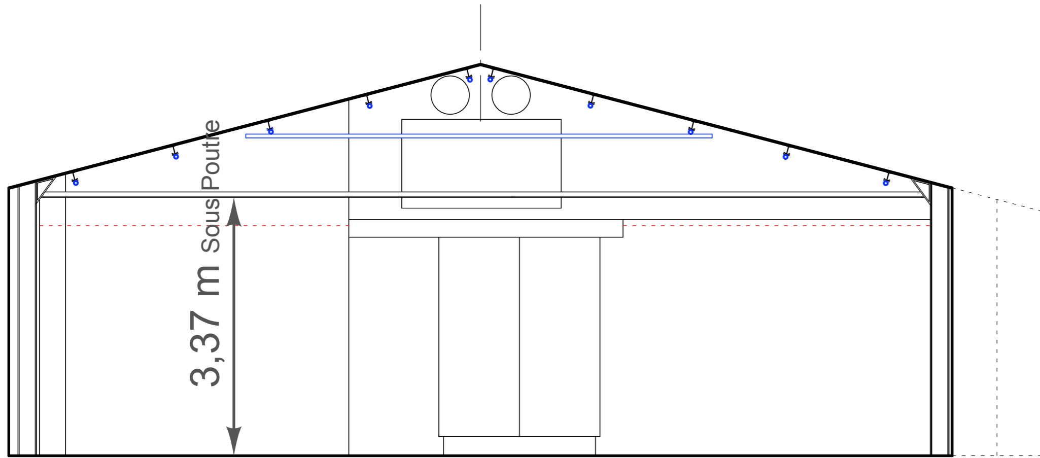
Coupe 1
